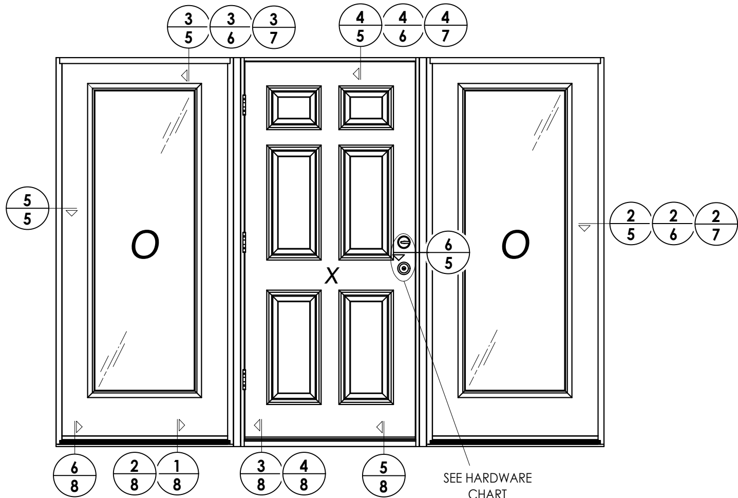
ELEVATION OXO
