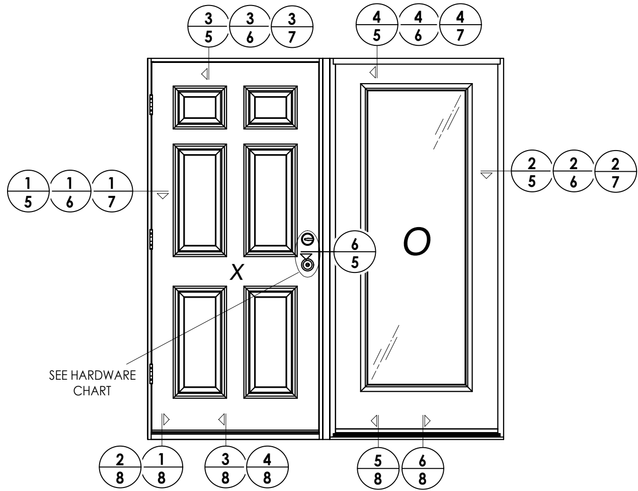
ELEVATION XO
